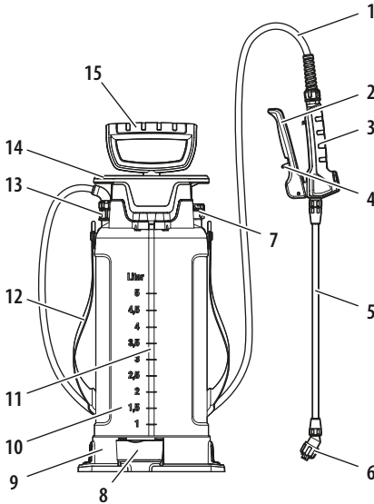
Telle des Drucksprüheräts
