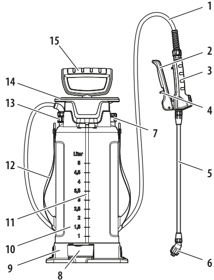
Onderdelen van de druksproeier
